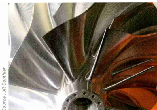
Turbine usinée sur une machine Starrag. (EMO 2017,
